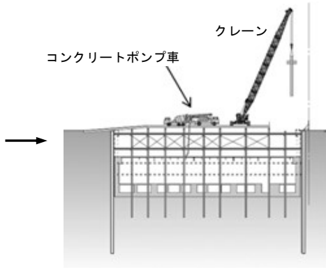
図 3-2-3-9(2) 施工概要（名城変電所）
